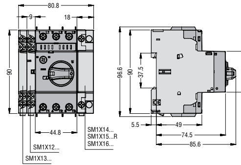
SM1R... mit seitlichen Hilfskontakten
