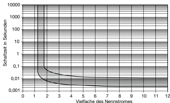
Kennlinien E2 (flink) für AC 50/60 Hz
