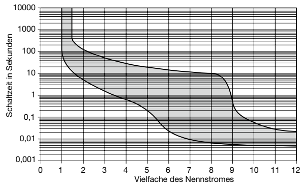
Kennlinien R2 (träge) für AC 50/60 Hz
