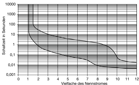
Kennlinien H2 (mittelträge) für AC 50/60 Hz
